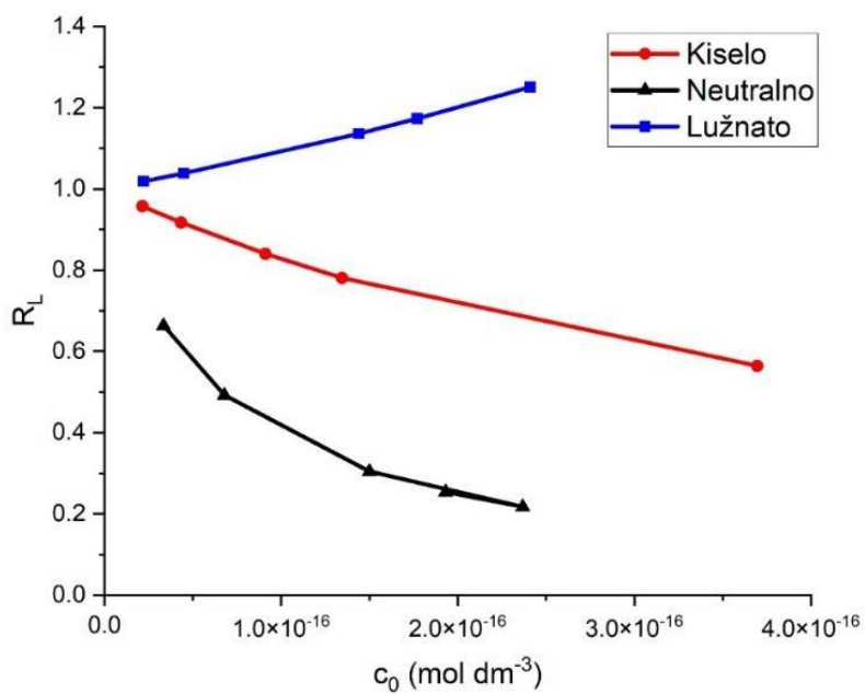
Slika 36. Ovisnost ravnotežnog parametra R_L o početnoj koncentraciji.
