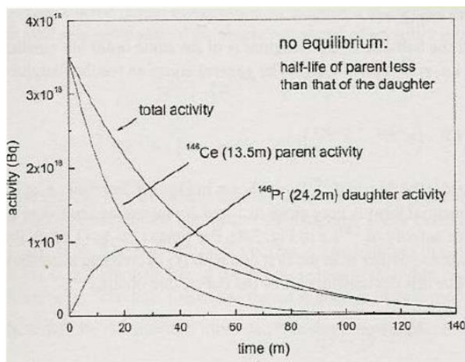
Slika 18. Grafički prikaz kad su jezgra roditelja ( 146 Ce) i jezgra kćeri ( 146 Pr) bez ravnoteže [17].
